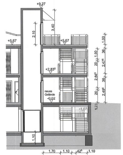
Schnitt C1-C1
