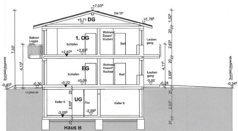
Schnitt A-A
