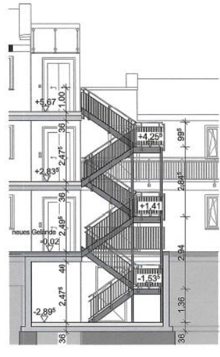
Schnitt C-C
