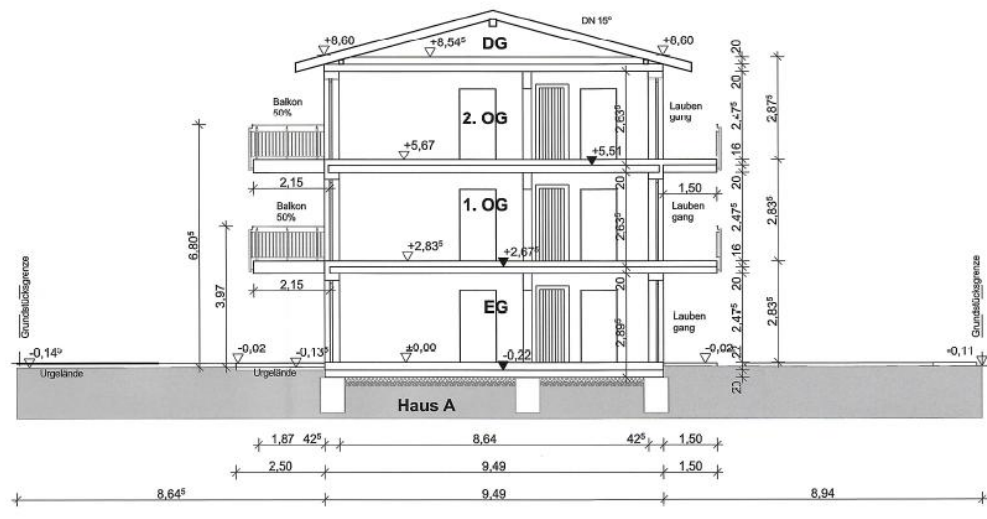
Schnitt B-B
