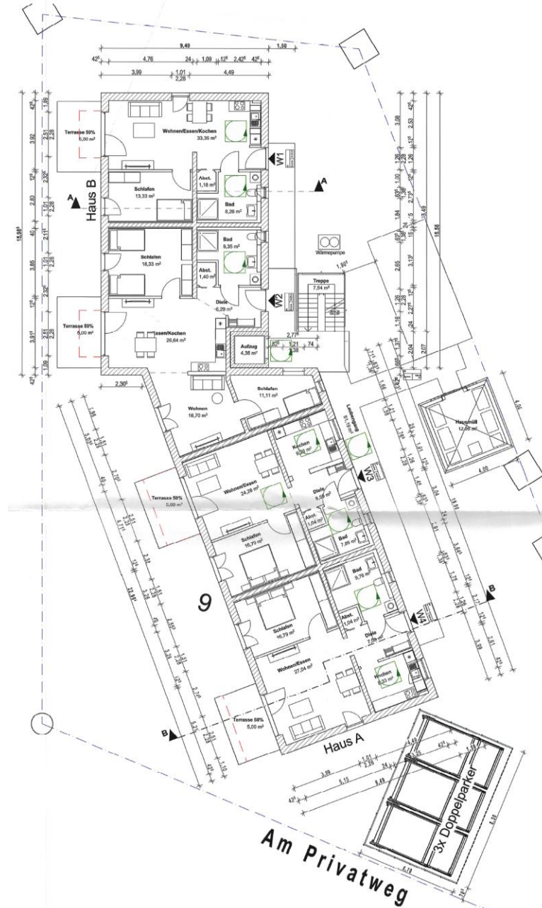
Grundriss EG
