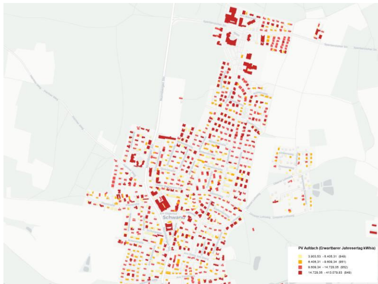
Solarpotenzialuntersuchung PV-Aufdach Beispiel Schwand
