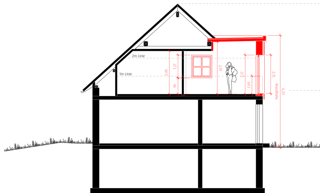
Schnitt _ 01 M 1 : 100
