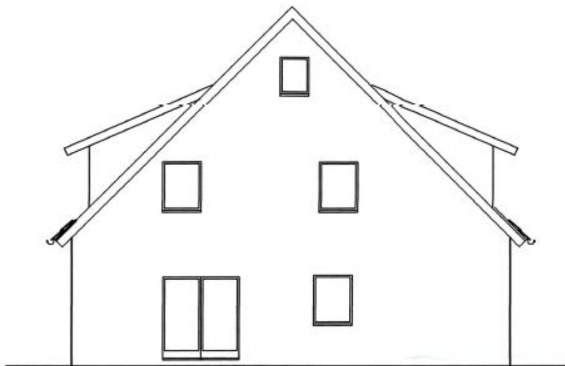
Ansicht Osten
