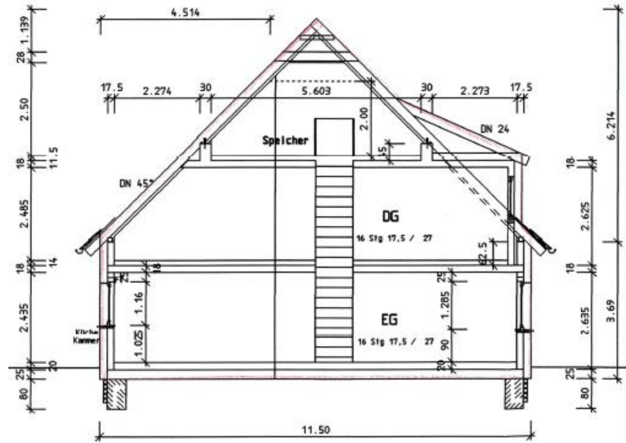
Schnitt
