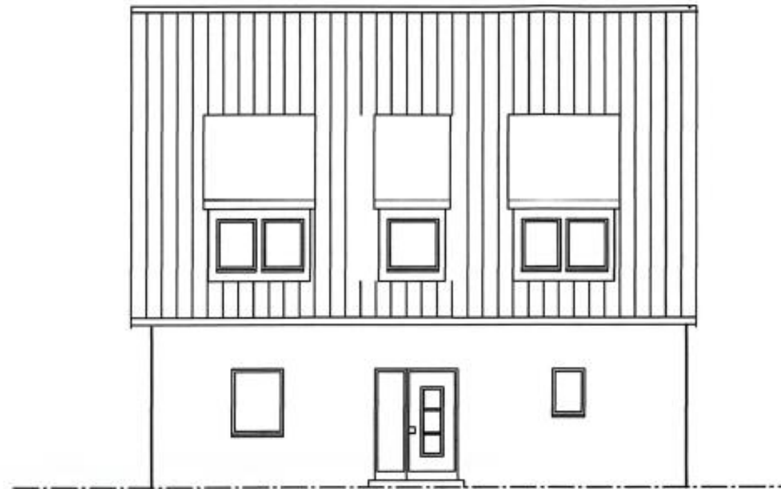
Ansicht Norden
