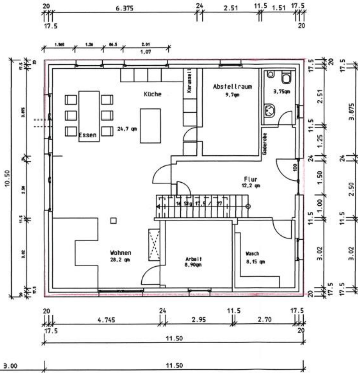
Erdgeschoss
