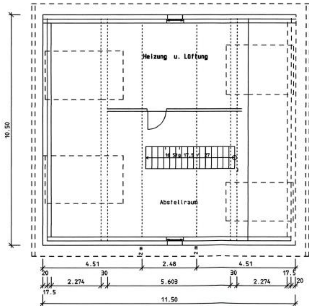
Spitzboden
