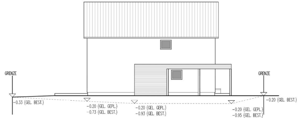
ANSICHT OST
