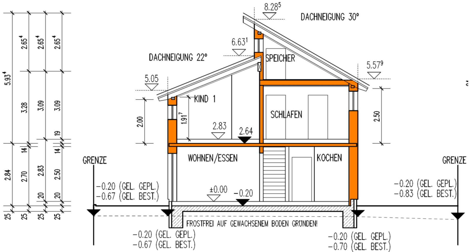
SNITT A-A
