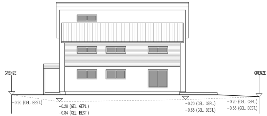
ANSICHT WEST
